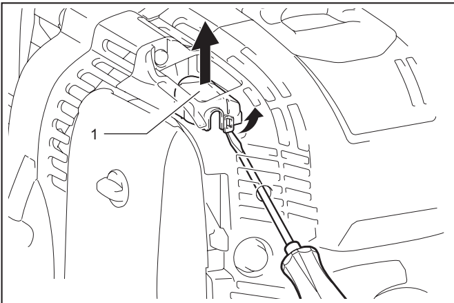
► 1. Kaasuttimen kansi
