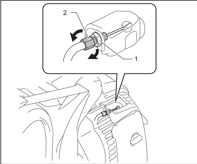
► 1. Kiinnitysmutteri 2. Kaapelin säätöpultti
